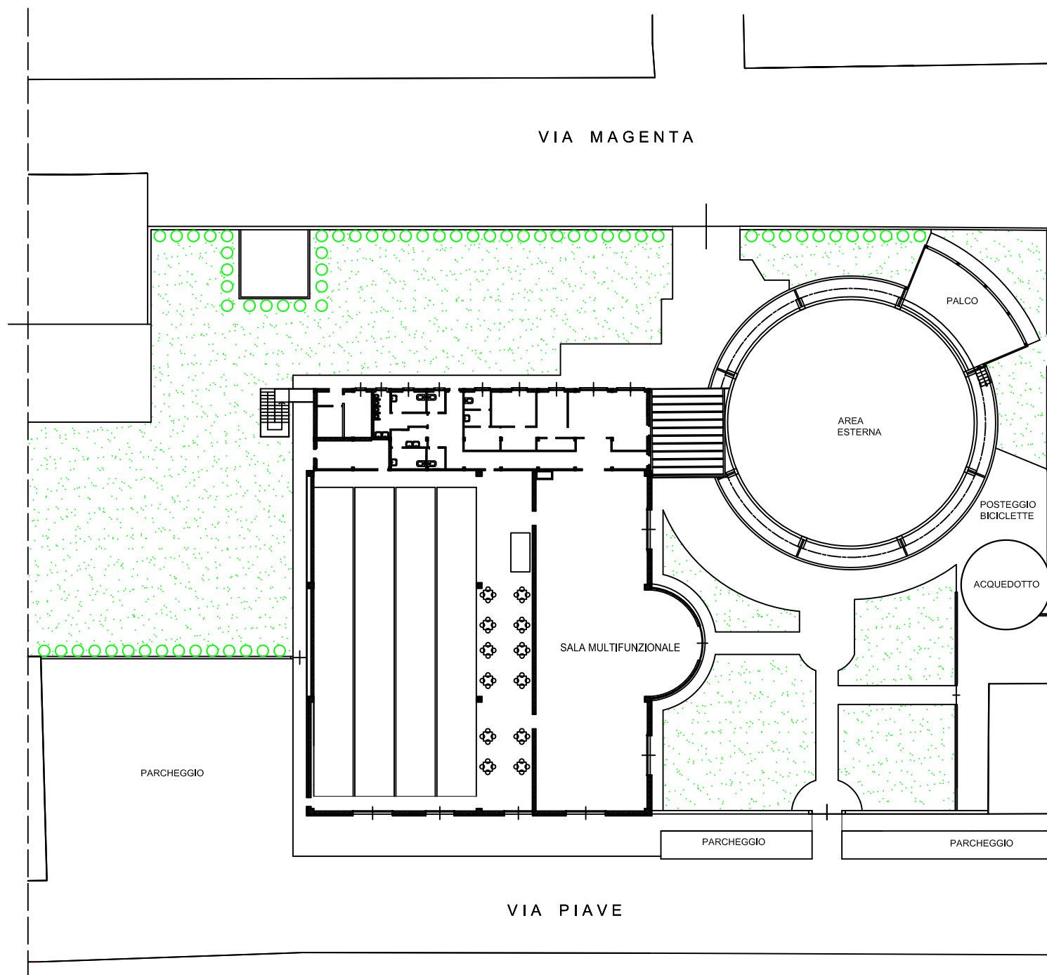
PLANIMETRIA N°2
